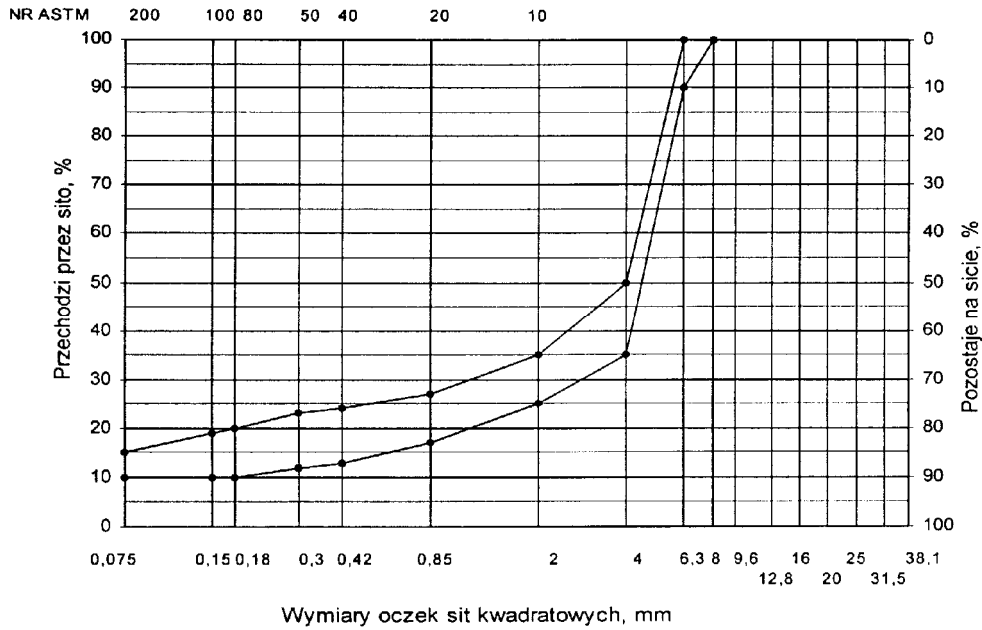
Rys. 3. Krzywe graniczne uziarnienia mieszanki mineralnej SMA od 0 do 6,3 mm do warstwy ściernalnej nawierzchni drogi o obciążeniu ruchem KR1 lub KR2
